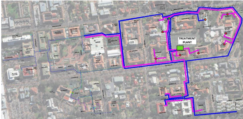
Figuur 8: Skematiese uitleg van siviele werke en pypleiding
